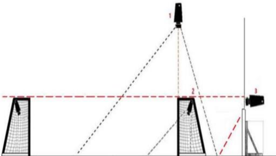
3. Схема расположения камер над воротами, за воротами и в воротах (вид сбоку):
